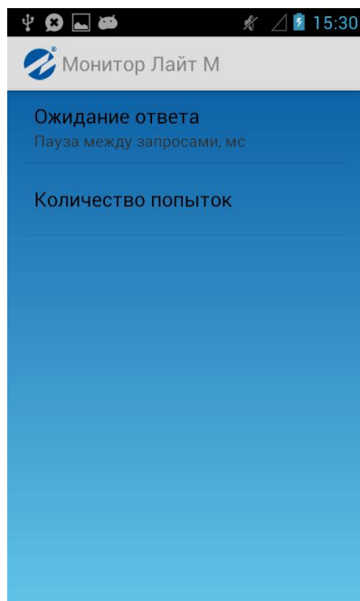
Рис. 20. Настройки приложения.
