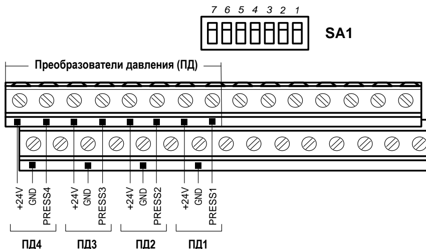
Рис.30. Обозначение коммутационных элементов подключения ПД.
