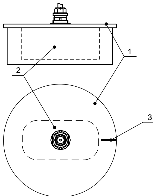
1 – крышка; 2 – датчик уровня; 3 – риска для установки по потоку.
