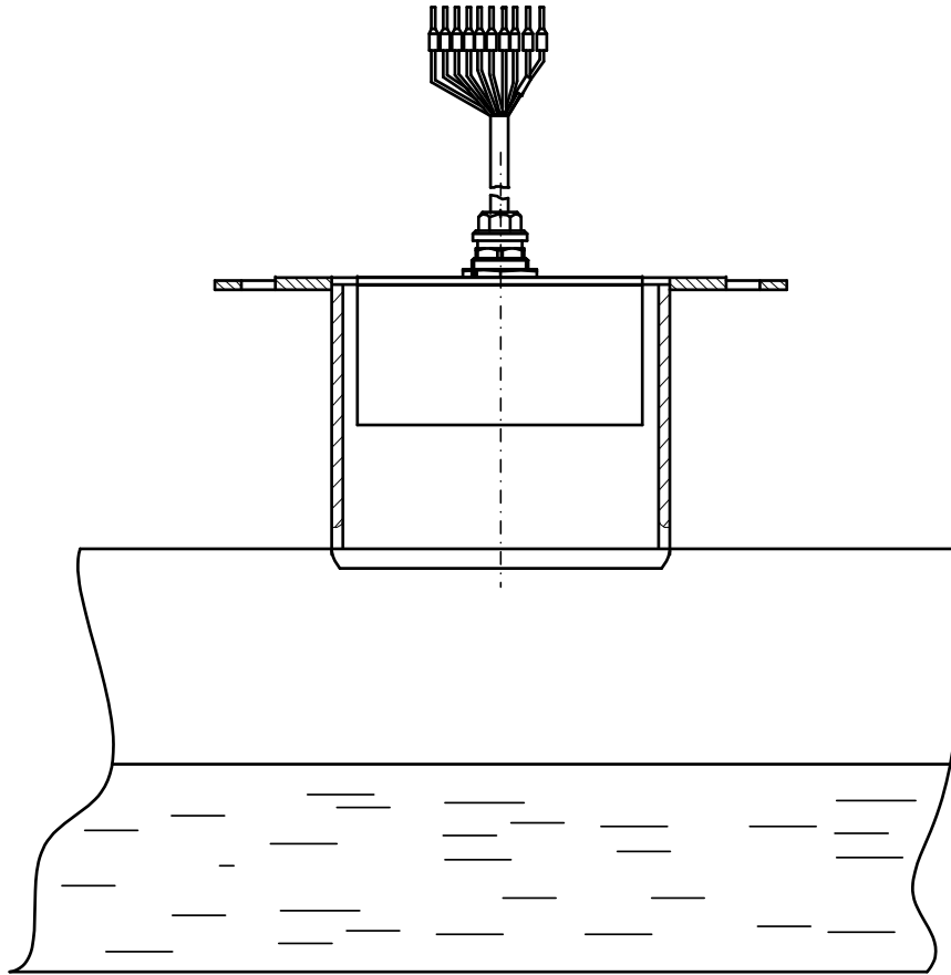
Рис.А.6. Монтаж АС-111-013 с помощью установочного патрубка.
